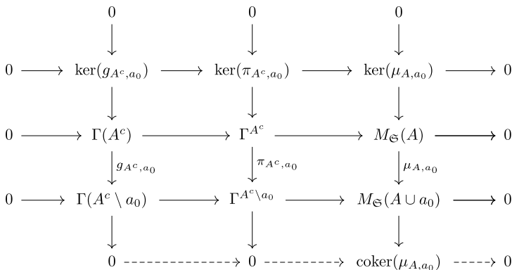
Fig. 14. Diagram for the proof of Lemma 9.11.
